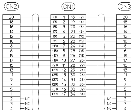
配線図
