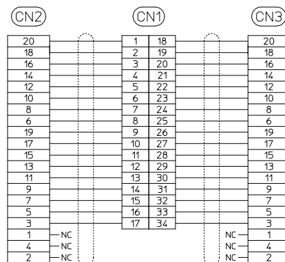
配線図
