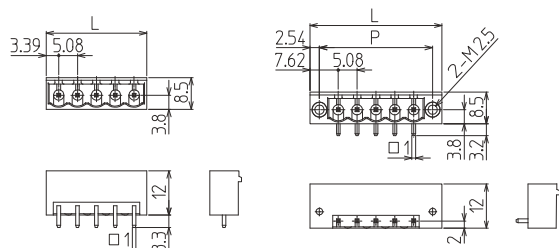
RK508B-□P コンタクトピン: ストレート
