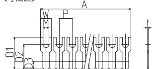
〔寸法図〕
