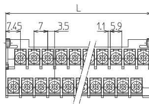
〔寸法図〕
