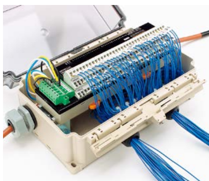
CC-Linkターミナル取付け例
