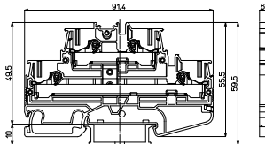
VTXW-4/2-PE
