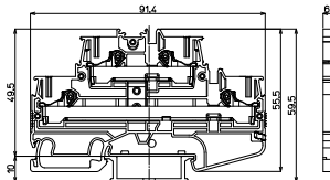
VTXW-4/2
