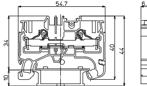
VTX-4/2
