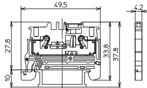
VTX-2/2-PE
