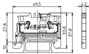
VTX-2/2
