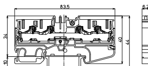
VTX-4/4-PE
