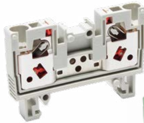
VTZ-4/2 質量 約11g 標準価格 128円/個 (税抜・販売単位:100)
