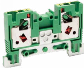
VTZ-4/2-PE 質量 約15g 標準価格 395円/個 (税抜・販売単位:20)
