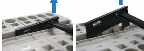
① 取外し用の角穴に適合 工具を差込み持ち上げる
