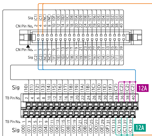
結線図 (TOP VIEW)
