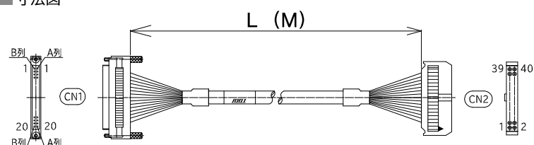
■寸法図
