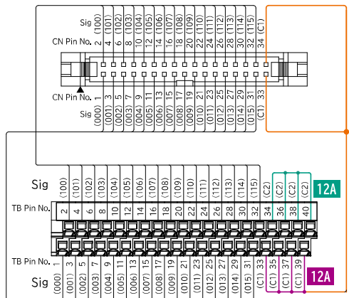
結線図 (TOP VIEW)
