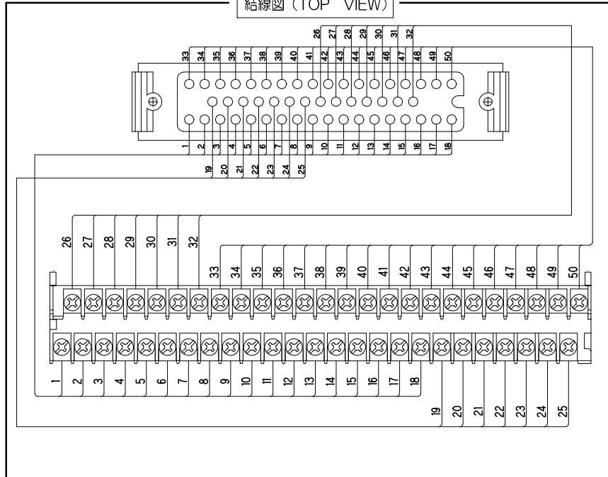
結線図 (TOP VIEW)
